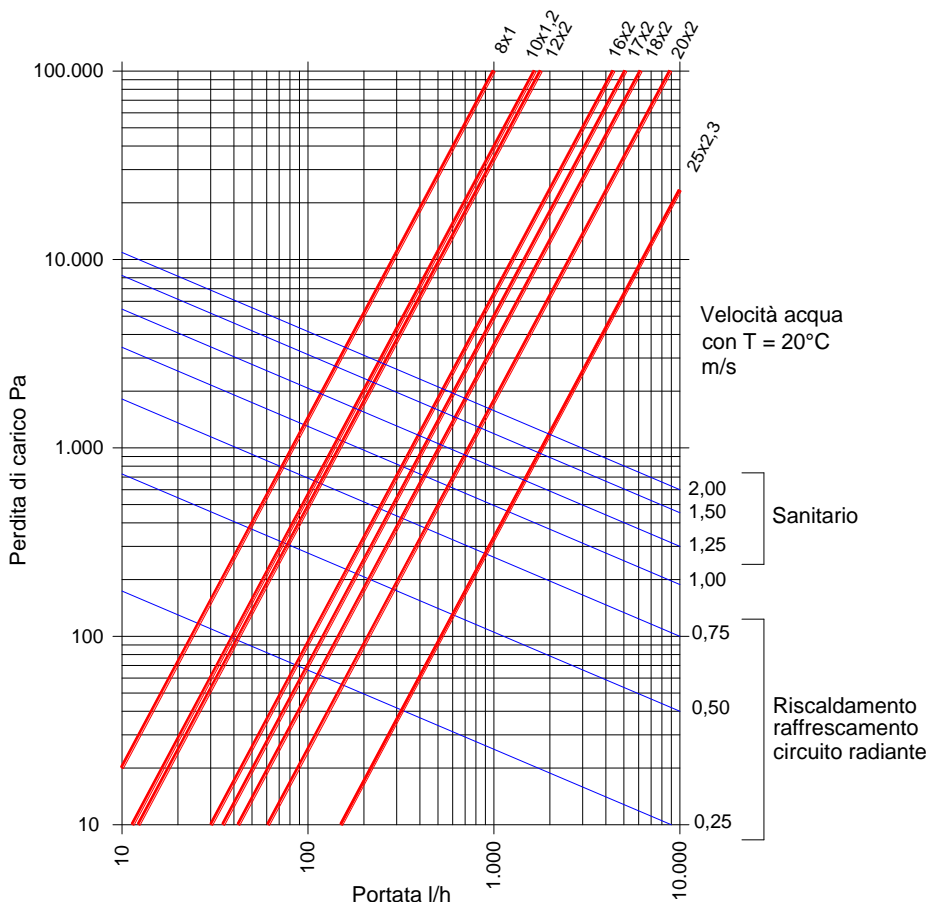
Grafico 4 – Perdite di carico nel tubo RBM KILMA-FLEX PE-Xc
